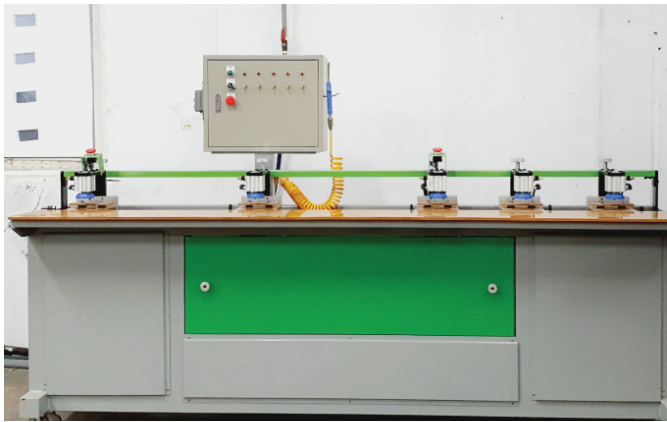
5축 경첩 보링기(유도보링장치)
